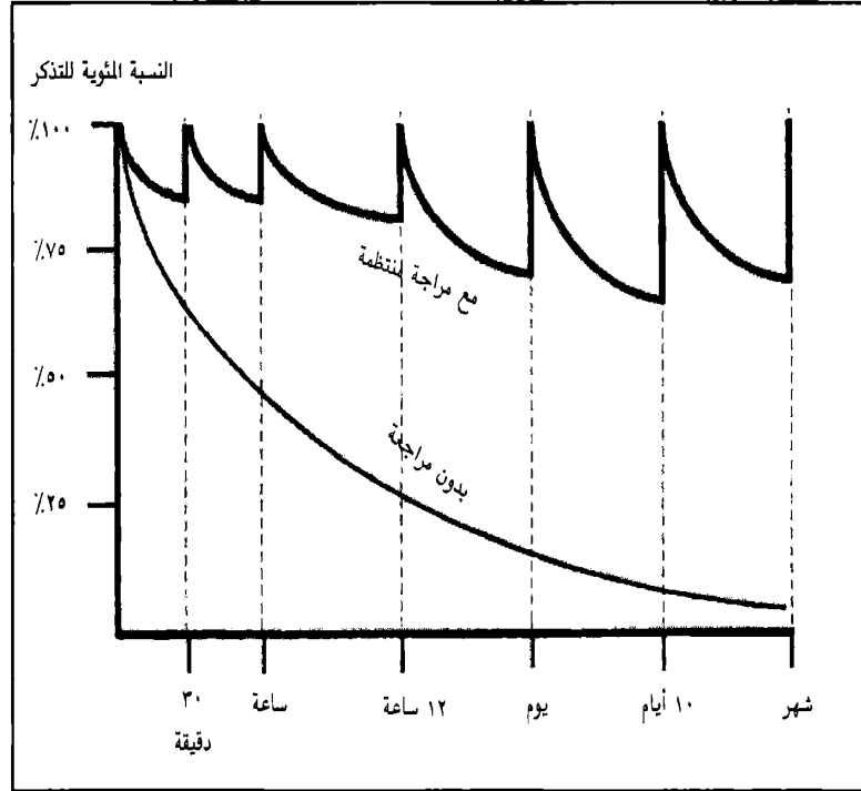
الشكل رقم ٦ تأثير المراجعة على التذكر
